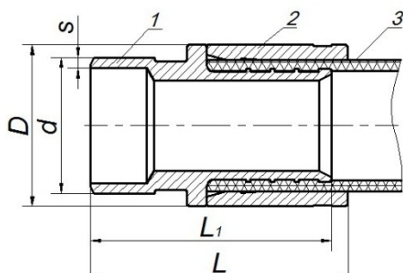
Рис. 6. Переход на сварное соединение с монтажной гильзой для труб ТВЭЛ-ПЭКС (Изопэкс)
