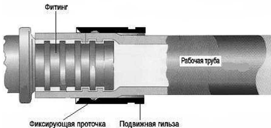
Рис. 21. Пресс соединение
