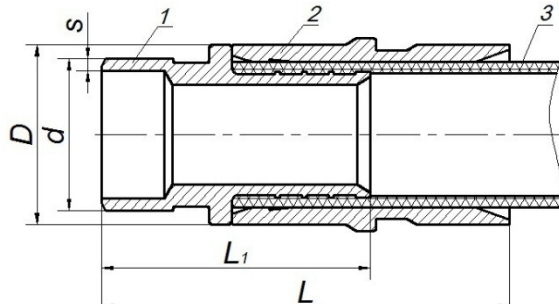
Рис. 7. Переход на сварное соединение с монтажной гильзой для труб ТВЭЛ-ПЭКС-К (Изопэкс-К)
